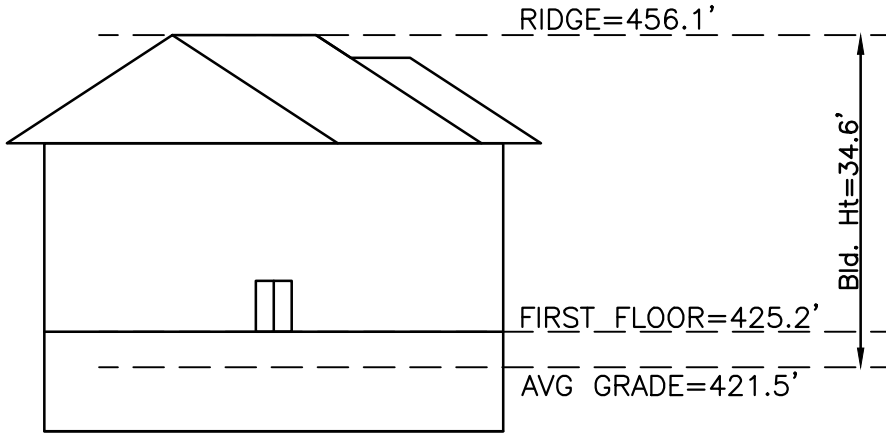
FRONT ELEVATION (N.T.S.)
