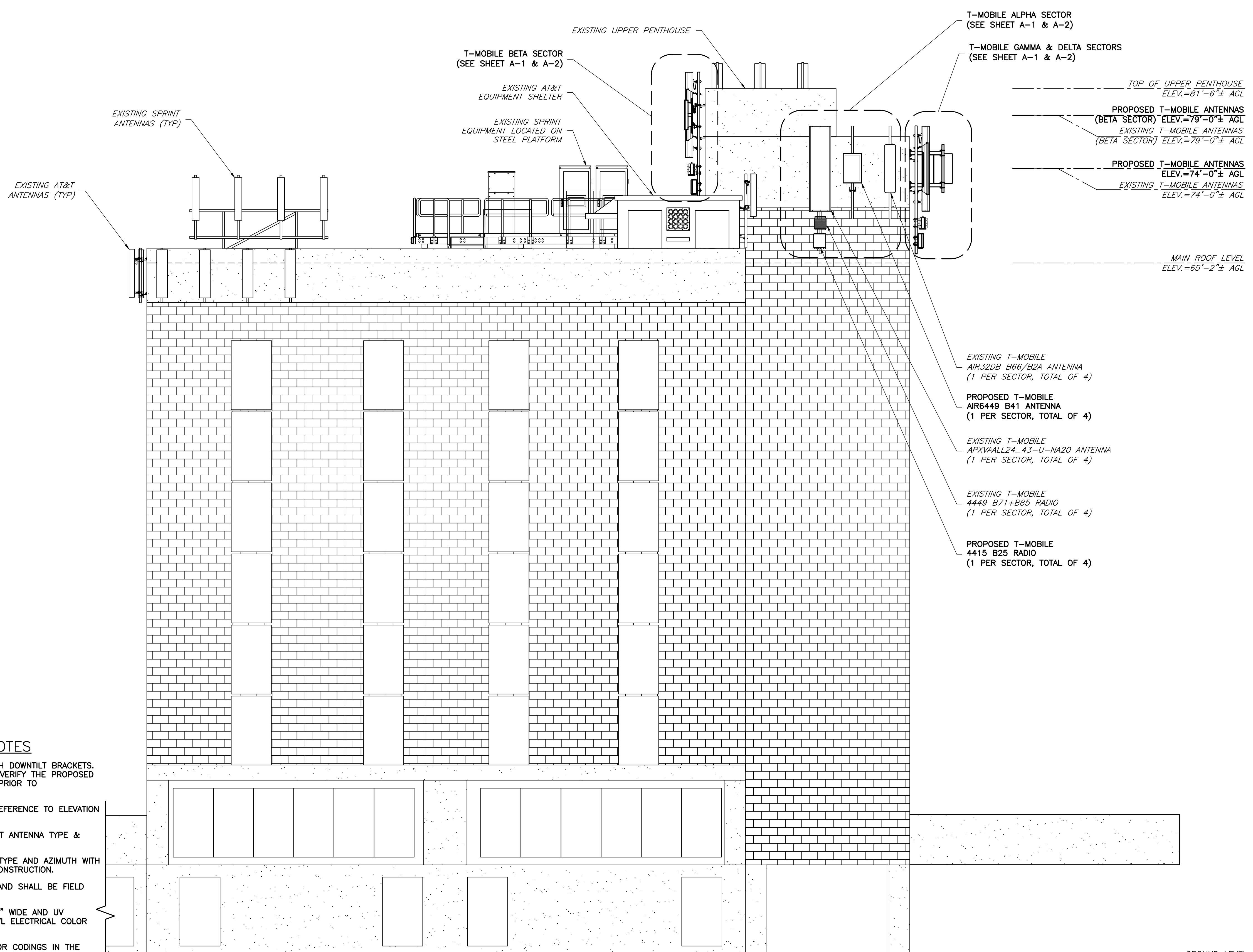
1 EAST ELEVATION SCALE: 1" = 5' (22X34) SCALE: 1" = 10' (11X17)
