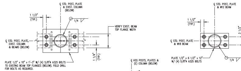
DETAIL A-A.
