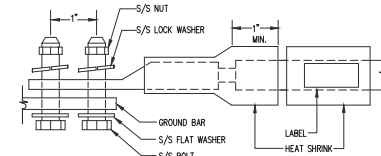
GROUND BAR ISOMETRIC SCALE: N.T.S.
