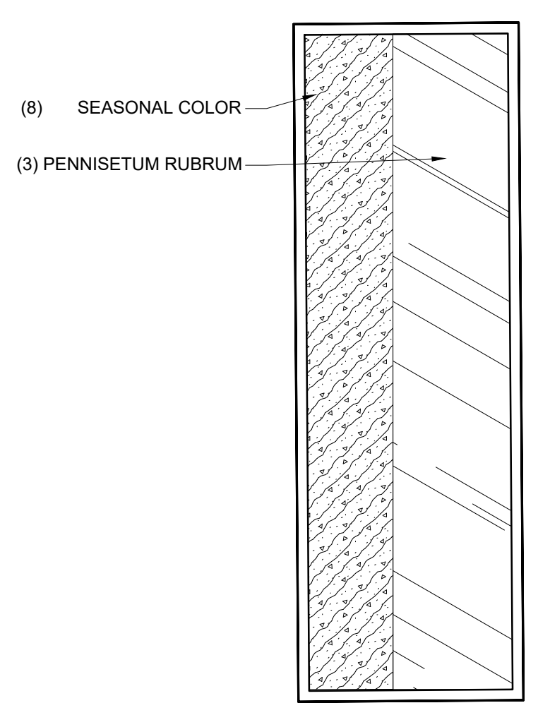
4 PLANTER TYPE 2 PLAN L6.03 Scale: 1" = 1'-0"
